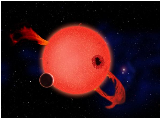
Рис. 1. Планета, вращающаяся вокруг красного карлика, в представлении художника. Рисунок David A. Aguilar с сайта universetoday.com . Все изображения с http://elementy.ru/novosti_nauki/432603
