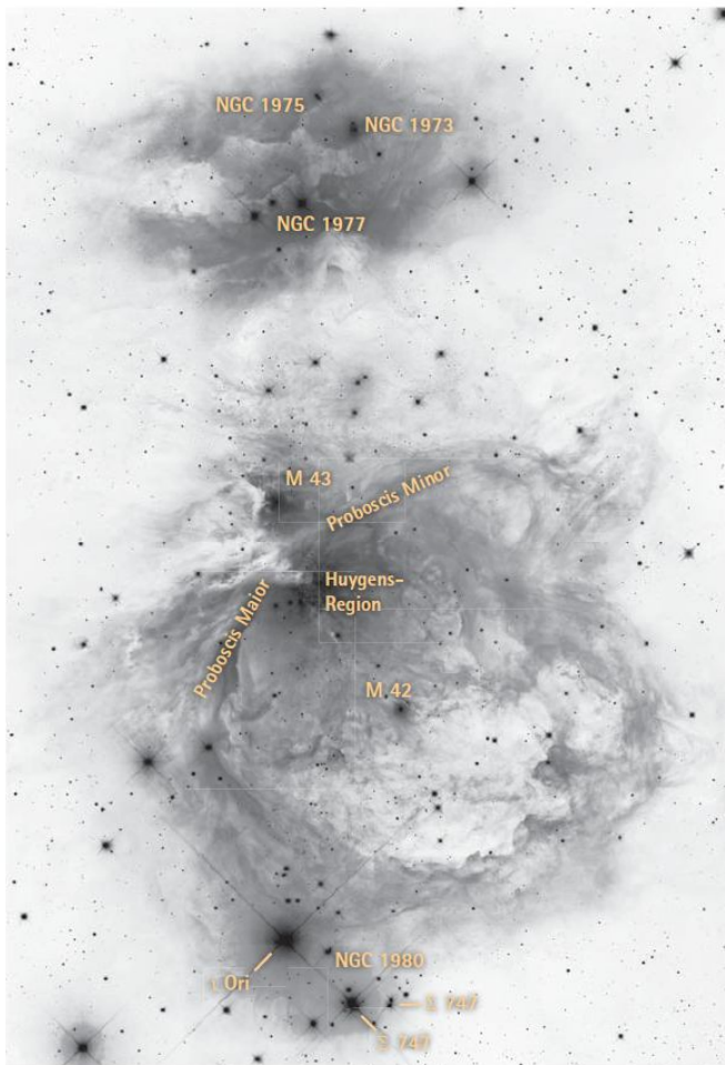
Объекты в M42. Guide 9.0
