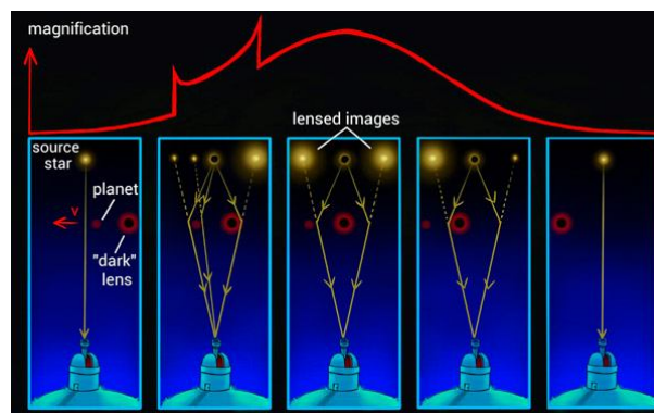
Рис. 2. Схематическое изображение события микролинзирования и изменения кривой блеска. Свет фоновой звезды усиливается, когда она оказывается на одной оси с близлежащей звездой. Если рядом со второй звездой есть планета, то образуется дополнительный пик на кривой блеска. Изображение с сайта theamateurrealist.com
