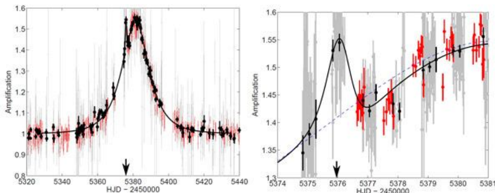
Рис. 4. Результаты наблюдений, которые позволили обнаружить новую экзопланету. По вертикальной оси отложено, во сколько раз увеличился блеск фоновой звезды, по горизонтальной — время в днях. Серые и черные точки — данные MOA, красные точки — данные OGLE. Черная линия — теоретически предсказанная кривая для этого события. Видно, что, хотя точек не очень много, они хорошо согласуются с теоретическим предсказанием. Черной стрелкой указан момент пика, соответствующего новой экзопланете. Справа это место показано крупнее. Синий пунктир — кривая блеска в модели без экзопланеты. Графики из обсуждаемой статьи
